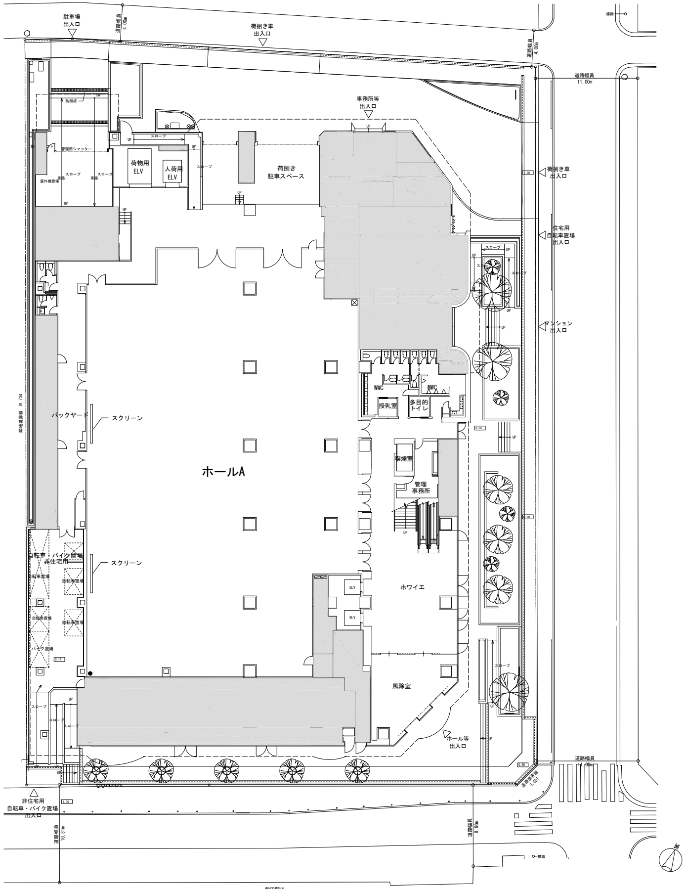
1階 平面図 1/400
