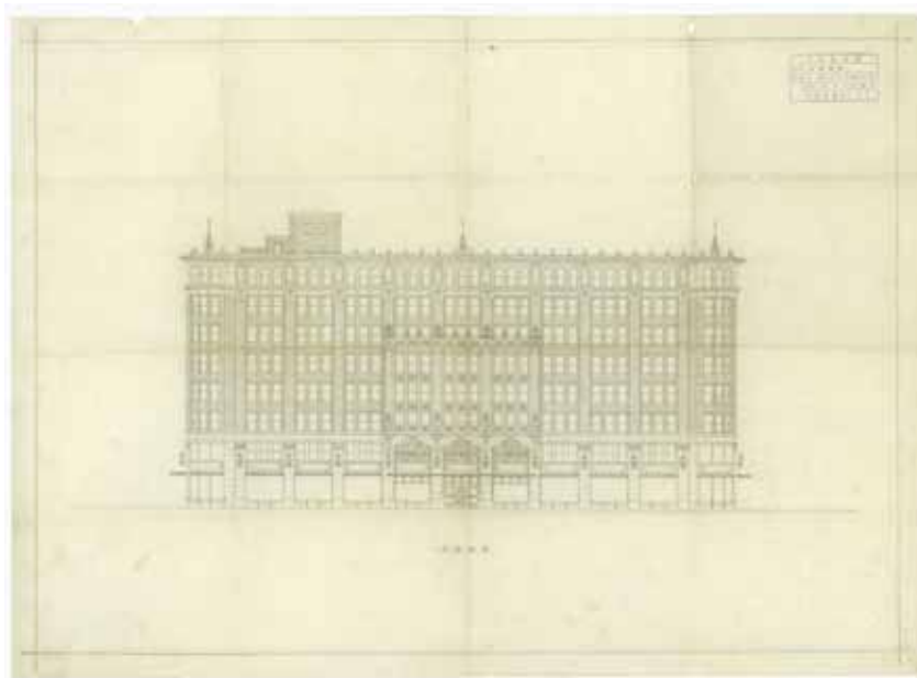
■日本生命館 正面建図 1/100 <AN.5071-14> 片岡事務所 京都工芸繊維大学美術工芸資料館所蔵
