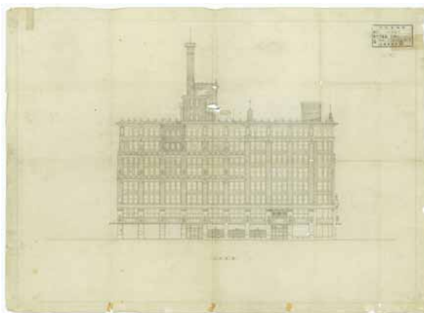
■日本生命館 左側建図 1/100 1931年 <AN.5071-15> 片岡事務所 京都工芸繊維大学美術工芸資料館所蔵
